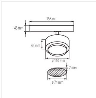
BTL 28W-930-W
