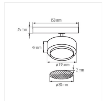
BTL 38W-940-B
