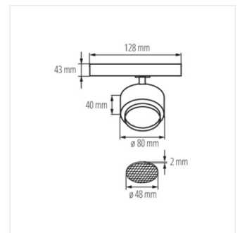
BTL 18W-940-B
