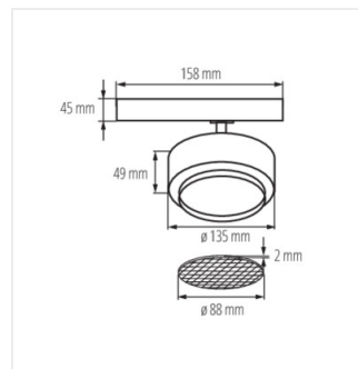
BTL 38W-940-W
