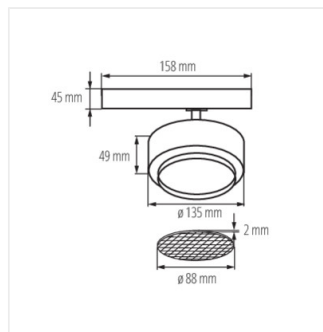
BTL 38W-930-B
