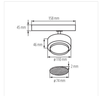
BTL 28W-940-B
