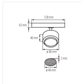
BTL 18W-940-W
