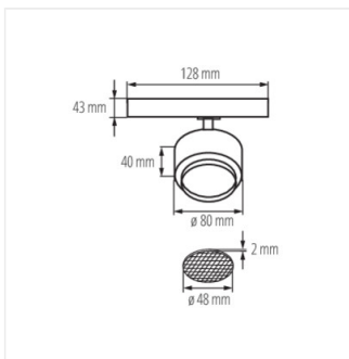
BTL 18W-930-W
