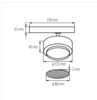
BTL 38W-930-W
