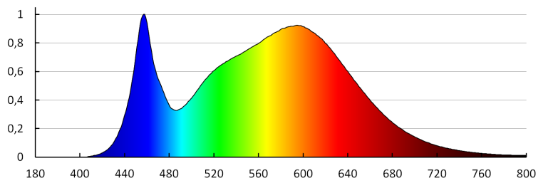
MILED0 (kat 31211) GU10 N LED 4W-NW / LDC (Polar)
